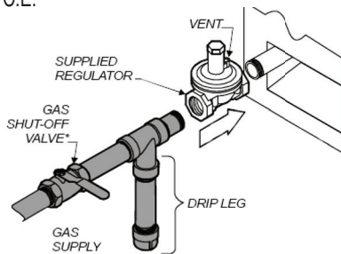
Connexion diagram
