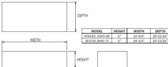
SPACER DIMENSIONS
